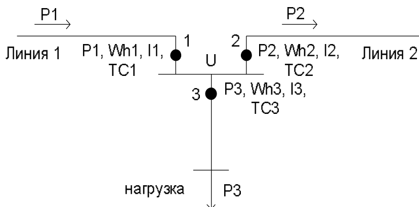
рис. 1 Участок схемы ЭЭС
