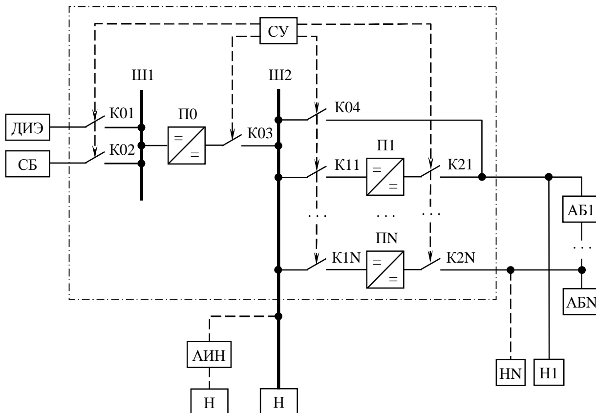
Рис. 2. Функциональная схема АСЭ с нестабилизированным выходным напряжением
