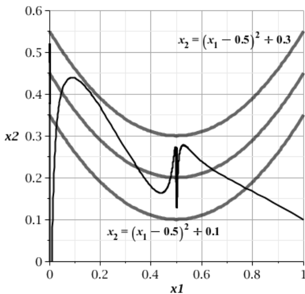
Рисунок 1. Фазовые траектории системы (6), два состояния равновесия – точки (0, 0.45 + 0.1 \sin t) , (0.5, 0.2 + 0.1 \sin t)
