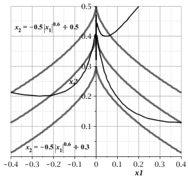
Рисунок 2. Фазовые траектории системы (6), одно состояние равновесия – точка (0, 0.4 + 0.1 \sin t)
