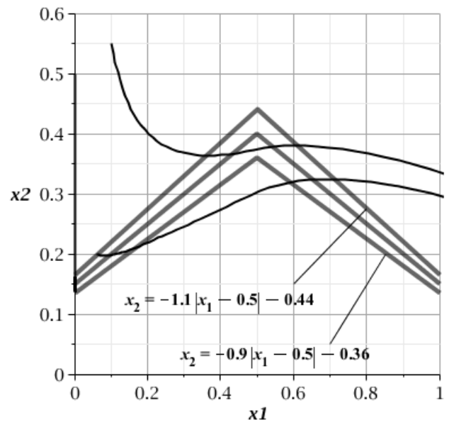
Рисунок 2. Одно состояние равновесия – точка (0, 0.15(1 + \sin t))
