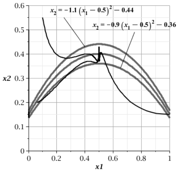
Рисунок 1. Два состояния равновесия – точки (0, 0.15(1 + \sin t)) , (0.5, 0.4(1 + \sin t))
