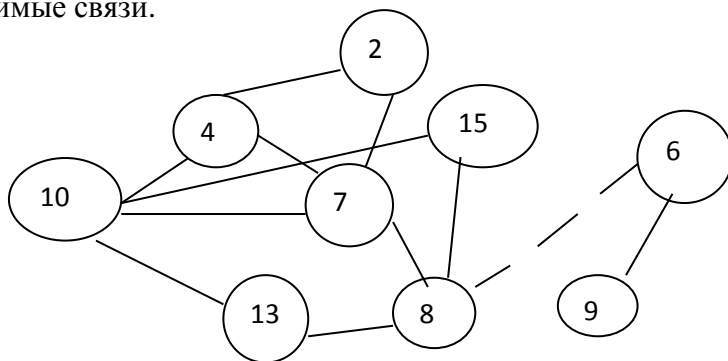
Рисунок 1. Корреляционная плеяда подростков – мальчиков
