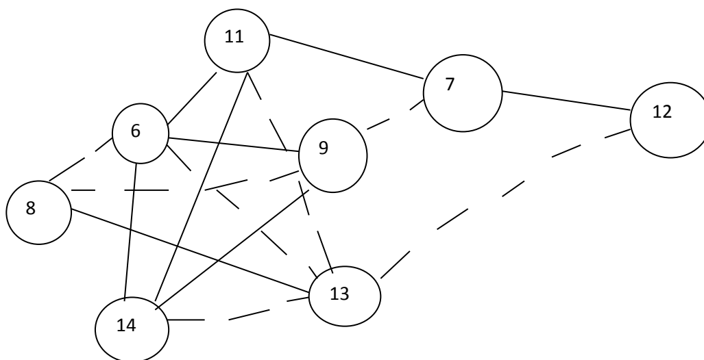
Рисунок 2. Корреляционная плеяда подростков – девочек
