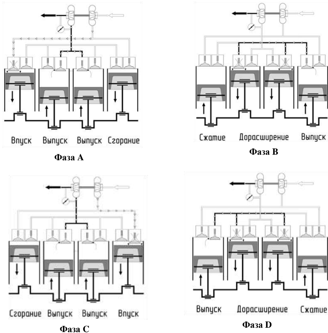
Рис. 1. Фазы рабочего цикла.
