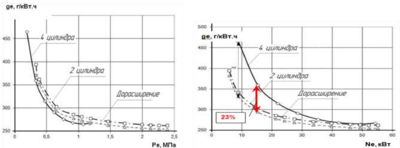
Рис. 2. Нагрузочные характеристики двигателя ВАЗ, n=4000 \text{ мин}^{-1}
