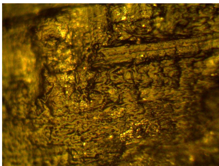
Рис. 2. Микроструктура композиционного образца ТРГ-полиэтилен (концентрация измельченного ТРГ - 10% по массе, без глицерина), увеличение 200 крат.
