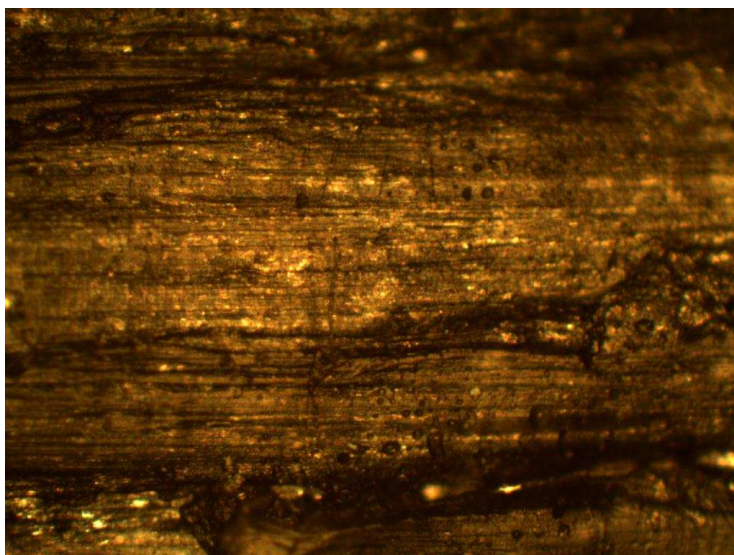
Рис. 1. Микроструктура композиционного образца ТРГ-полиэтилен (концентрация измельченного ТРГ - 10% и глицерина - 9% по массе), увеличение 100 крат.
