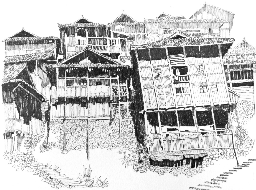
Рис. 5. Висячие стойки и нависающие карнизы
