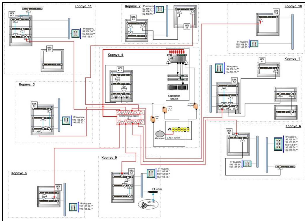
Рис. 2. Структурная схема топологии локальной вычислительной сети МБК
