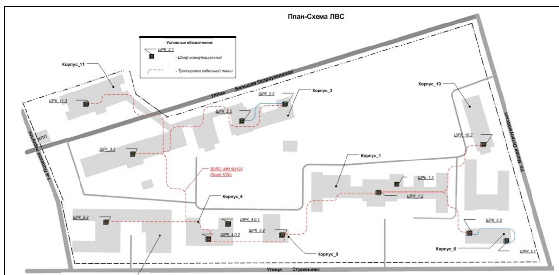
Рис. 1. Структурная план-схема ЛВС МБК на примере ГБУЗ «ГКБ № 5 ДЗМ»
