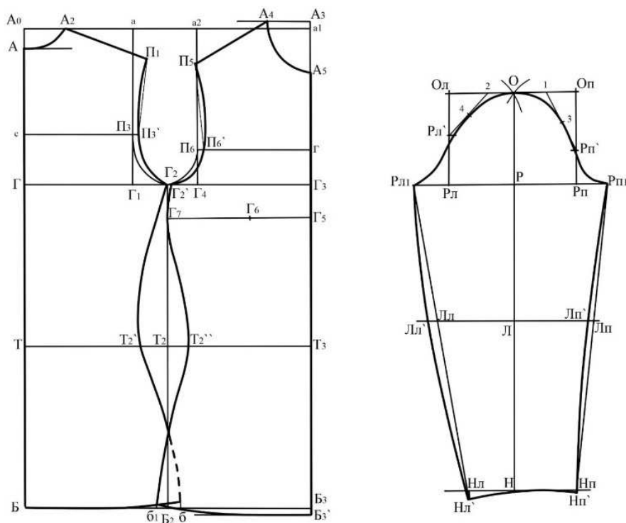
Рис. 2. Чертеж конструкции трикотажного изделия из полотен II и III групп растяжимости
