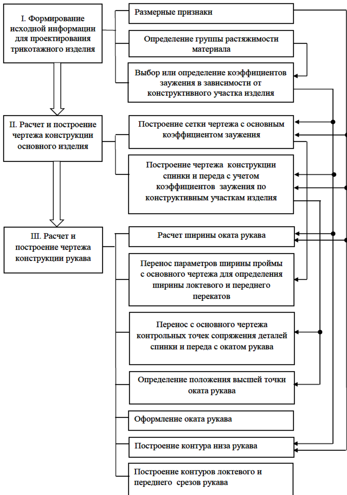
Рис. 1. Этапы построения базовой конструкции втачного рукава в зауженных трикотажных изделиях
